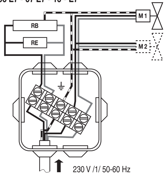
MRE 75 - 110 - 135 FJ 06 E7 - 07 E7 - 10 - E7
